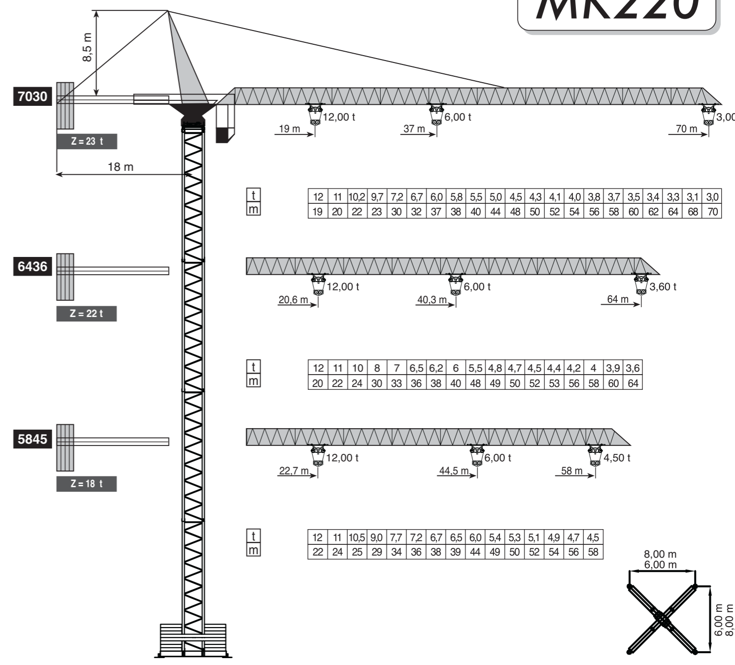
МАКСИМАЛЬНАЯ ВОЗМОЖНАЯ ВЫСОТА КРАНА С ПРИСТЕЖКОЙ – 200 МТ MT. 200 POSSIBLE MAX HEIGHT WITH ANCHORAGE FRAME
